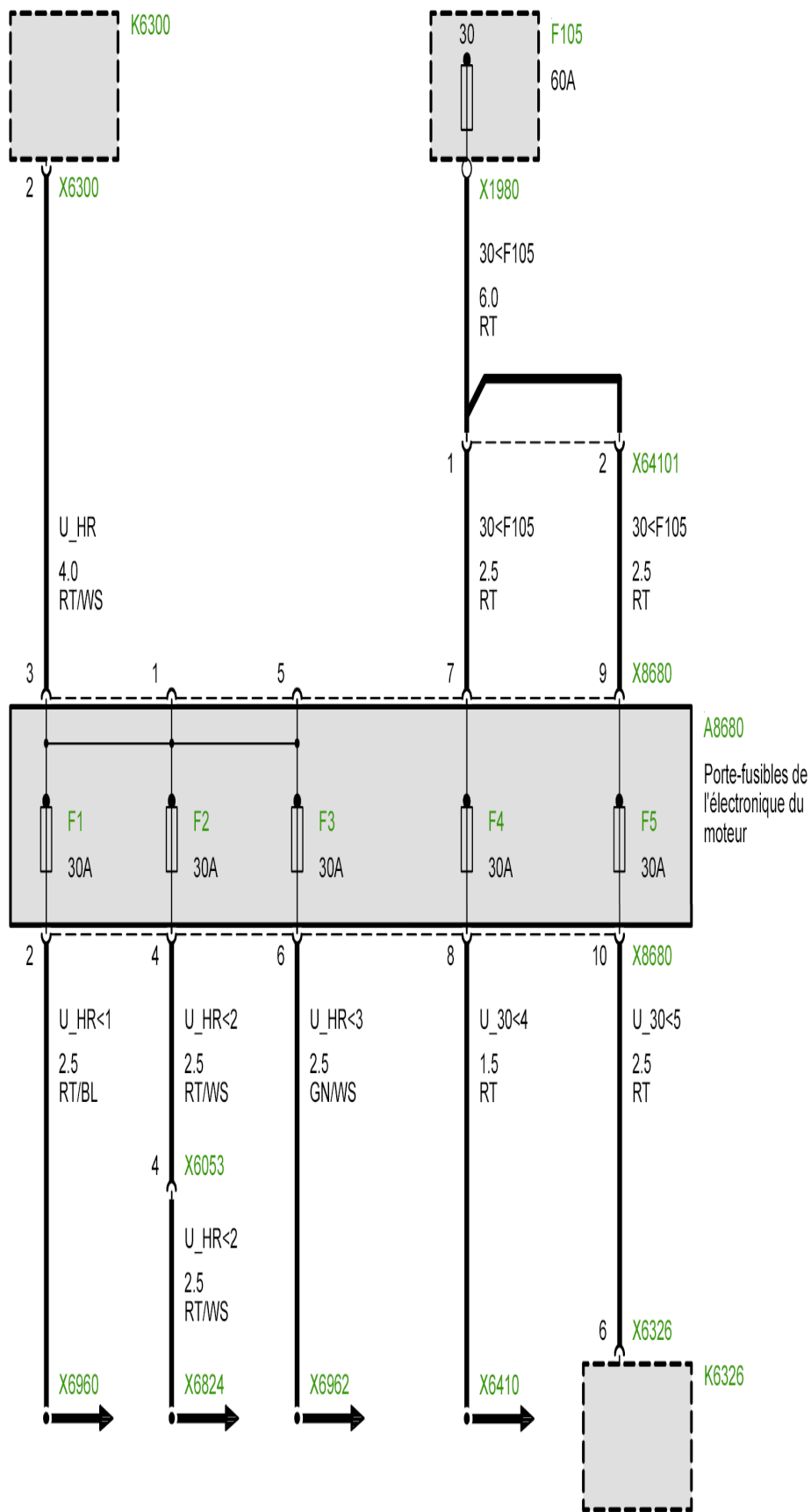
E53 A8680 Porte-fusibles de l'électronique du moteur
